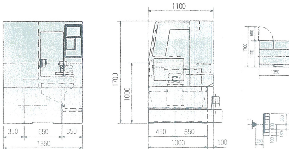
標準主要寸法図
